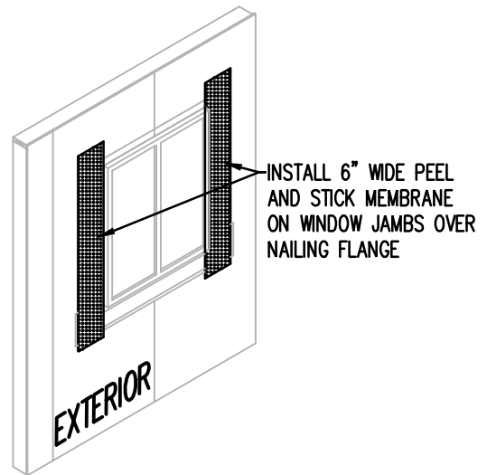
5 INSTALLATION OF JAMB MEMBRANE B-002 SCALE: N.T.S.
